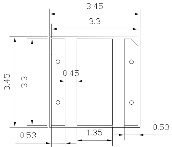
背面图
